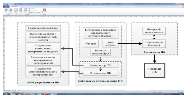
Рис. 1. Архитектура программного средства разработчика «SWDesigner».
