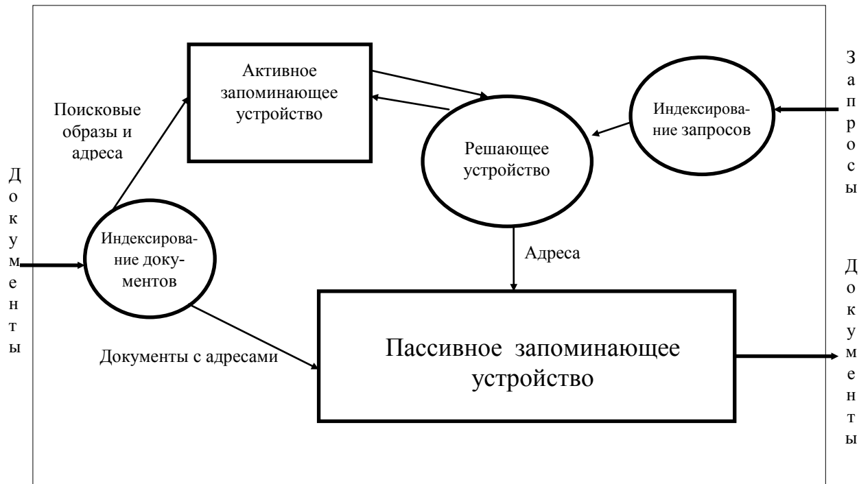
Рис. 9. Блок-схема информационно-поисковой системы
