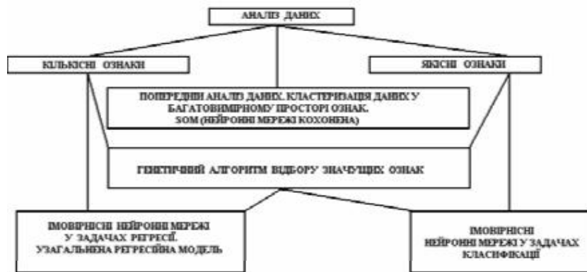
Рис. 4. Структура пакету аналізу даних BioStatNeuro
