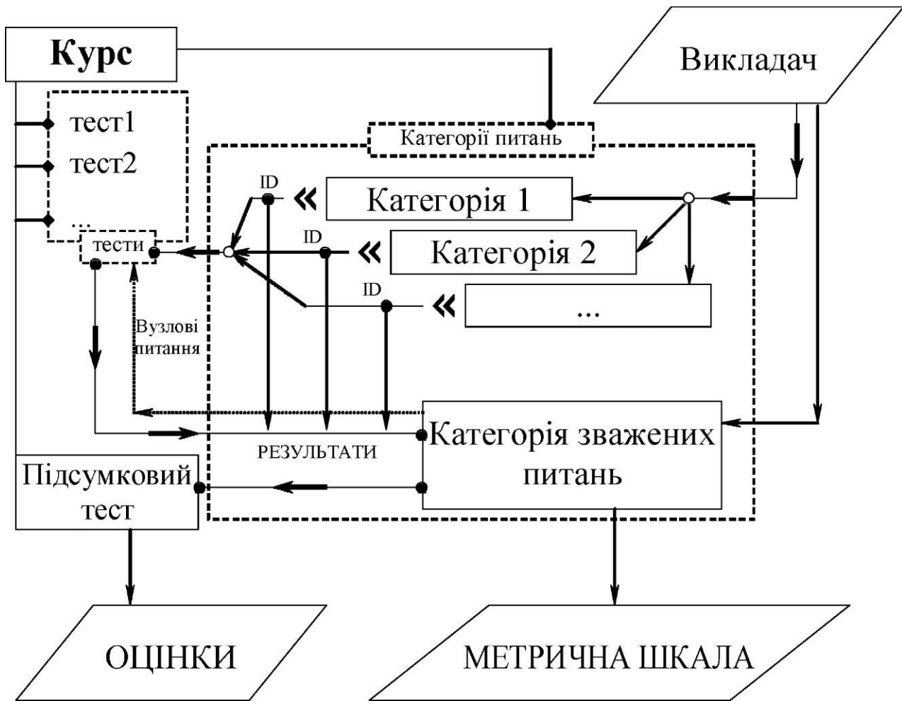
Рис.2. Блок-схема програми
