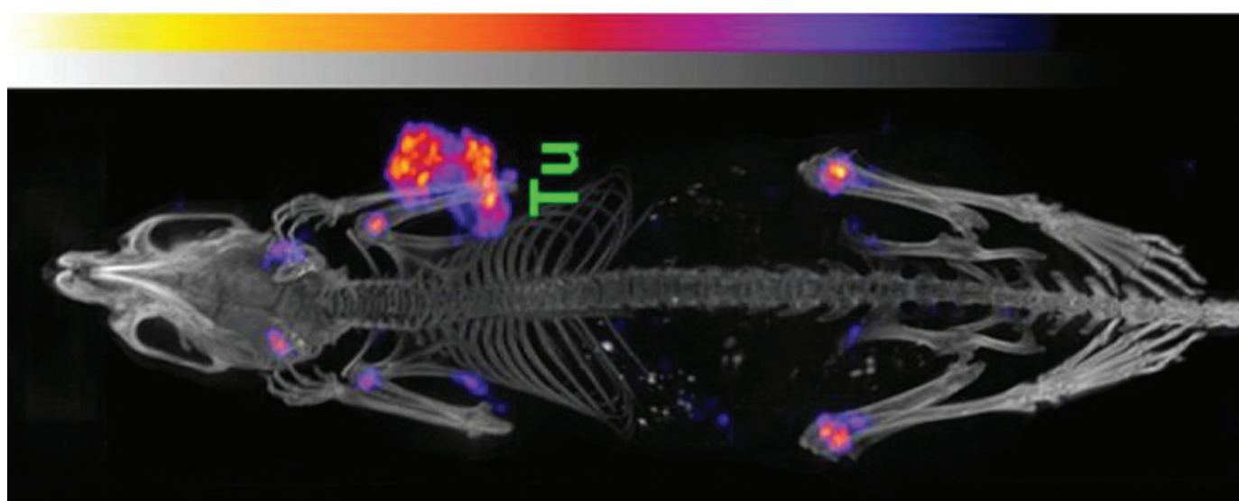
Рис. 5. ОФЕКЕТ/КТ зображення миші (М №5), що має підшкірний ксенотрансплант пухлини SKOV-3ір через 3 дні після введення ^{155}\text{Tb} -СНСЕ7 (4,2 МБк). Накопичення радіоактивності було виявлено в ксенотрансплантаті пухлини та в кістках (Tu = пухлина) [26].
