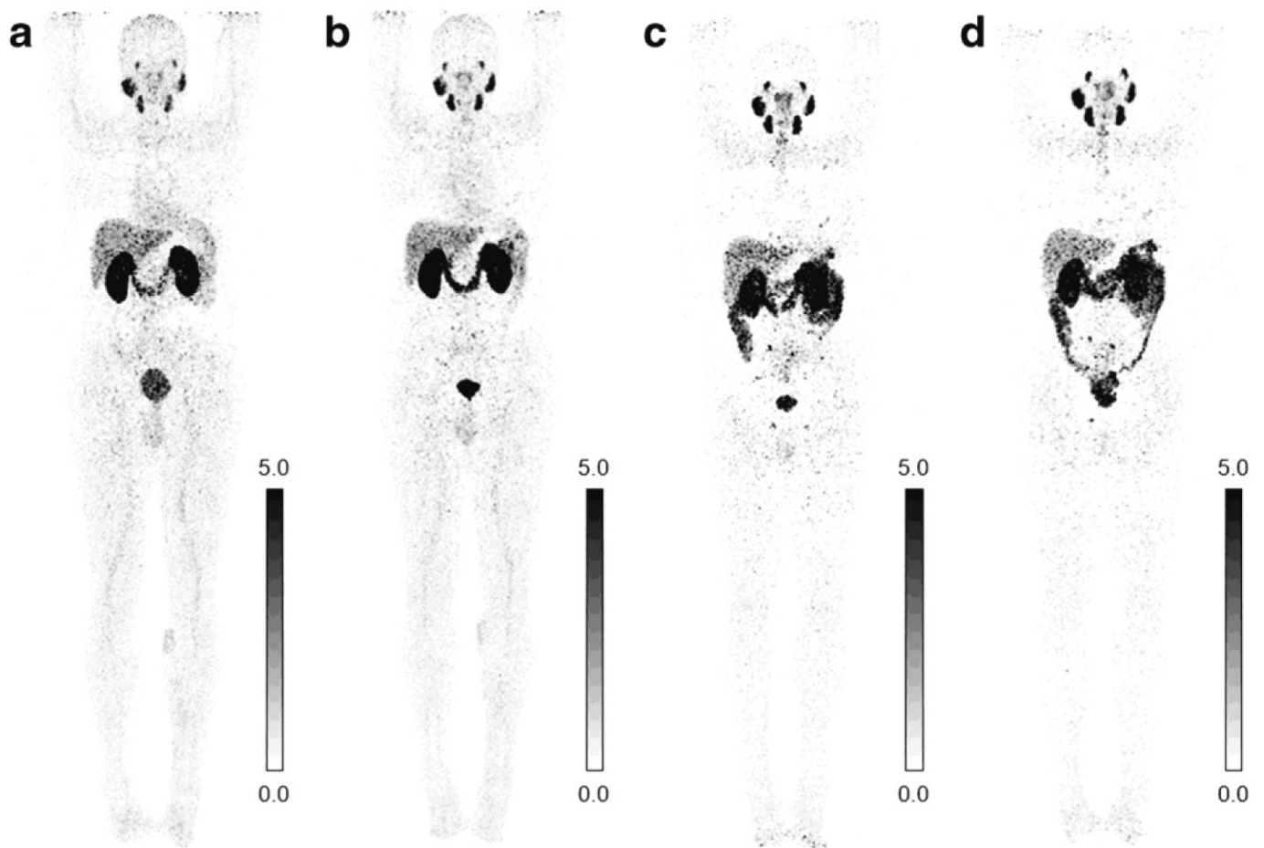
Рис. 2. Фізіологічний біорозподіл ^{152}\text{Tb} -ПСМА-617 на ПЕТ/КТ (MIP-зображеннях), отриманих за а. 50 хв, б. 2 год., с. 18,5 год., д. 25 год., відповідно після введення 140 МБк ^{152}\text{Tb} -ПСМА-617. Фізіологічне включення радіолінду спостерігається в басейнах слізних, привушних і підщелепних залозах, слизовій оболонки носоглотки, а також у печінці, селезінці та кишкового тракту. [45].
